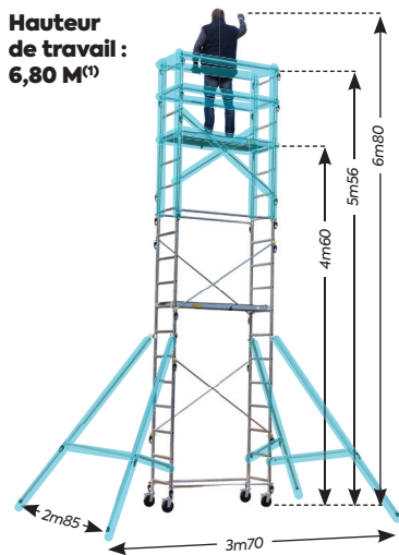
/// Rehausse QUAD'UP
