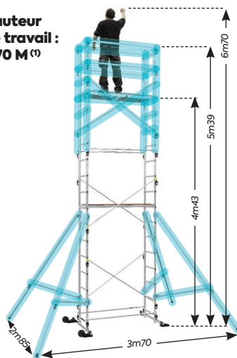
/// Rehausse TEK'UP
