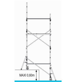
/// Fonction rattrapage de niveau
